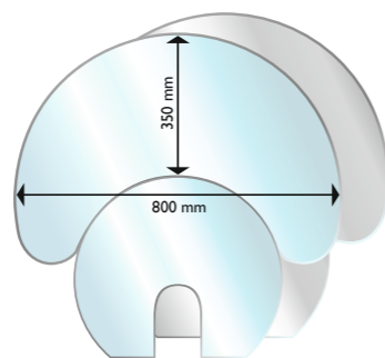
Halvmåne glasgulvplade Passer til Aduro 1.1-serien, 9-serien (undtagen 9.4) og 17-serien. Fås i gråt og klart glas.
